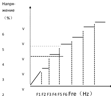
Рис 6-4 Полигональная линия Режим V/F
