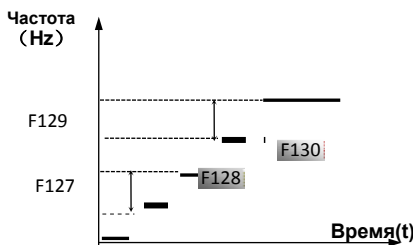
Рис. 6-2 Частота пропуска
