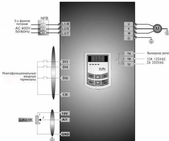
Рис. 5-3 Схема подключения 3
