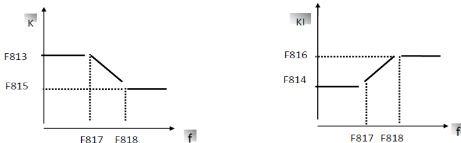
Рис. 6-22 параметр PID
