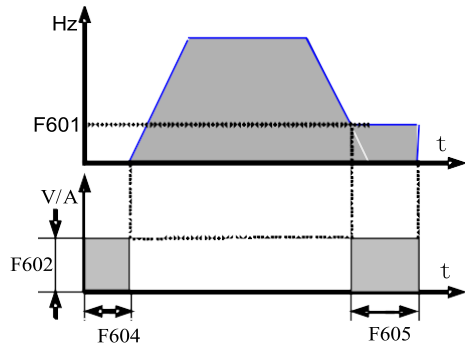
Рис. 6-19 DC торможение
