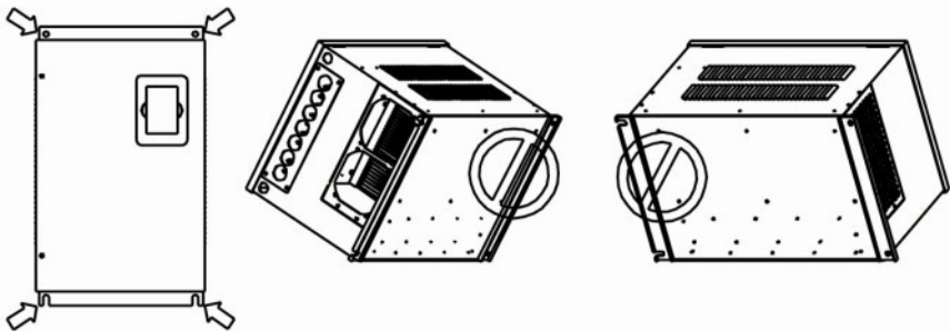
Рис. 1-2 Вертикальная установка
