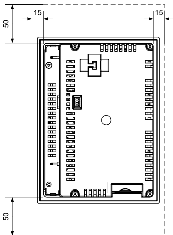
Рисунок 3-8 Зазоры при установке устройства НМИ
