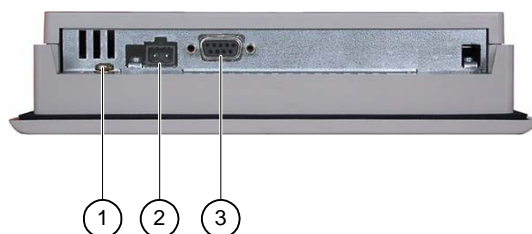
Рисунок 4-12 Интерфейсы устройства НМІ
