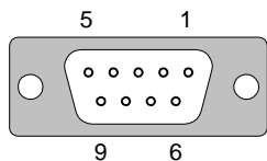
Рисунок 11-5 Назначение контактов интерфейса RS 485
