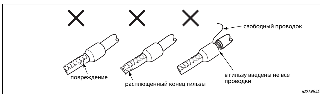
Рис. 3-9: Неправильно обжатая оконцовочная гильза
