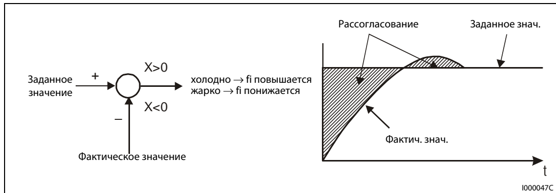
Рис. 6-122: Нагрев
