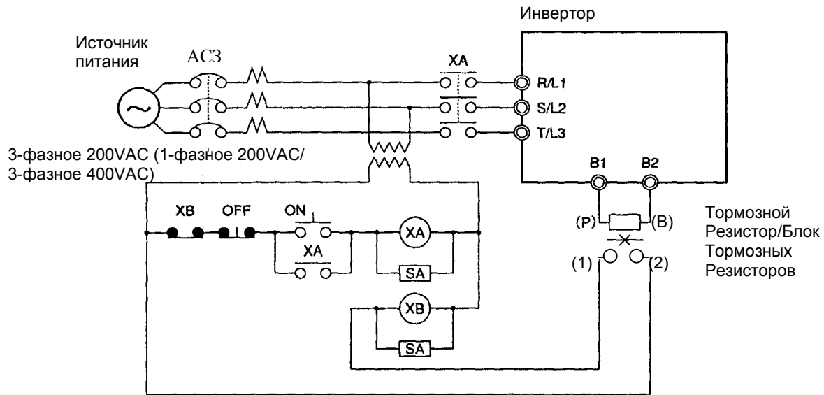
Контактные точки для терморазмыкателя Тормозного Резистора или внешнего термореле
