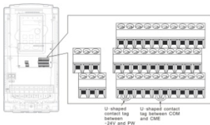
Рис. 3-7 U-образный контакт
