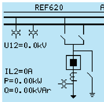
Рис. 25: Однолинейная схема с обозначениями ANSI
