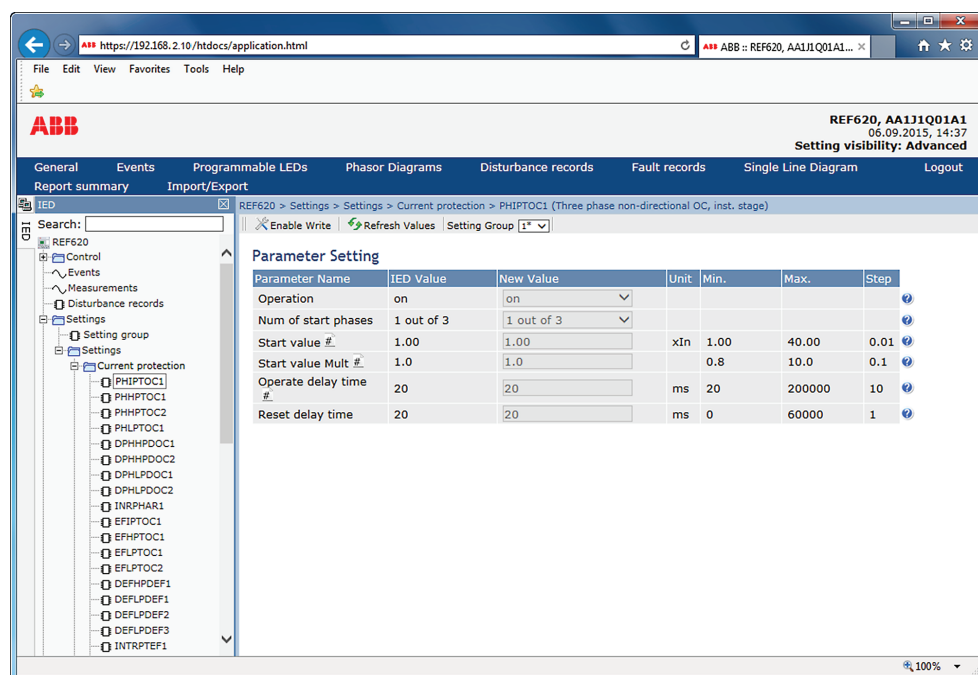
Рис. 7: Пример Веб-ИЧМ
