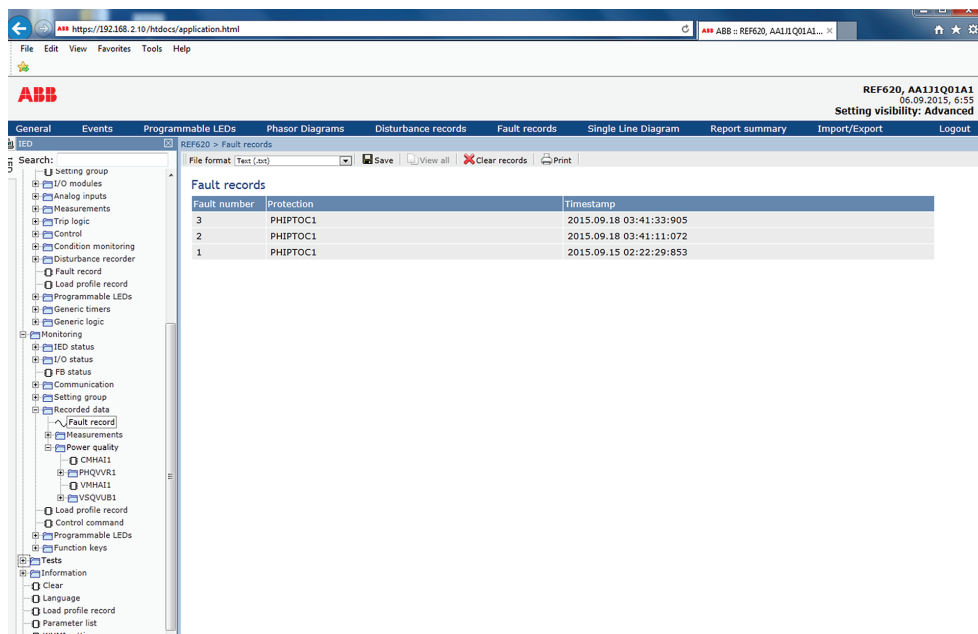
Рис. 63: Список записей аварий
