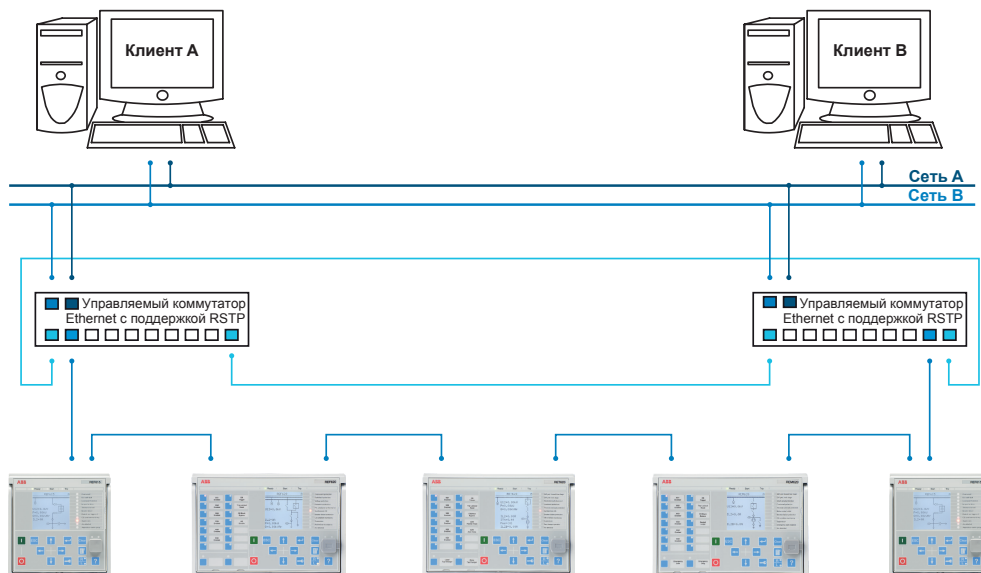
Рис. 8: Самовосстанавливающаяся кольцевая топология Ethernet
