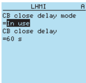
Рис. 96: Изменение режима выдержки времени на включение
