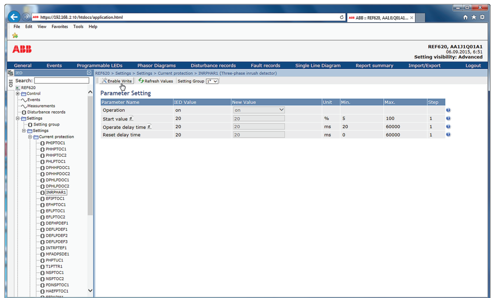
Рис. 39: Функциональный блок Вкл
