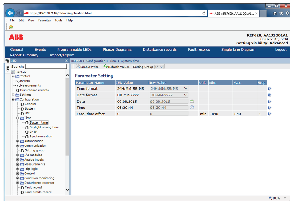
Рис. 36: Перемещение по меню веб-ИЧМ
