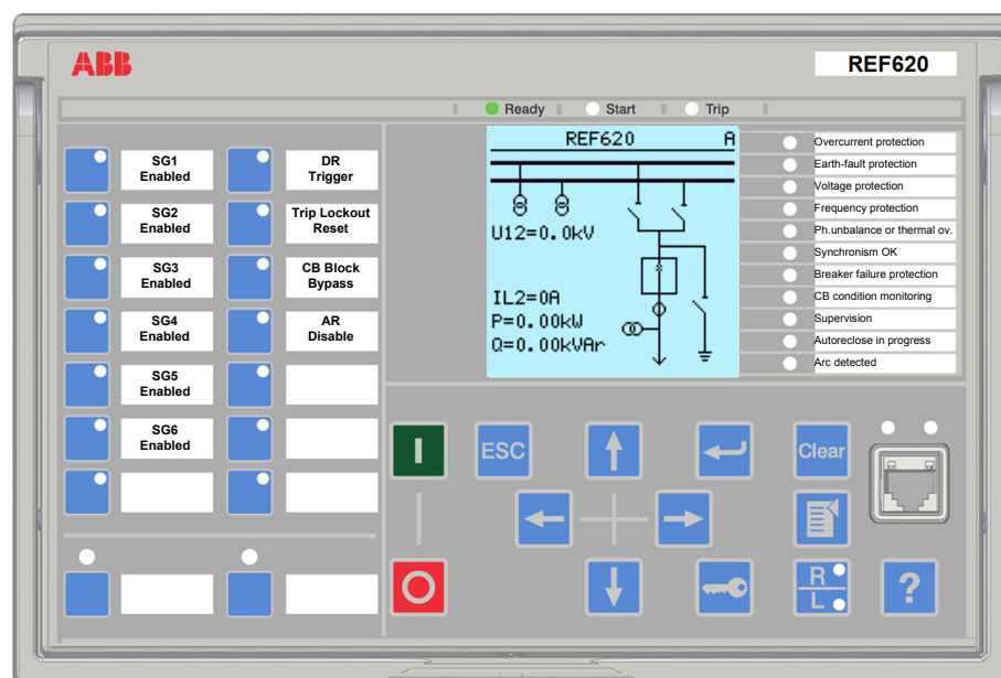
Рис. 2: Пример Локального ИЧМ
