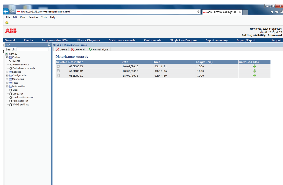
Рис. 55: Экран записей аварийных осциллограмм
