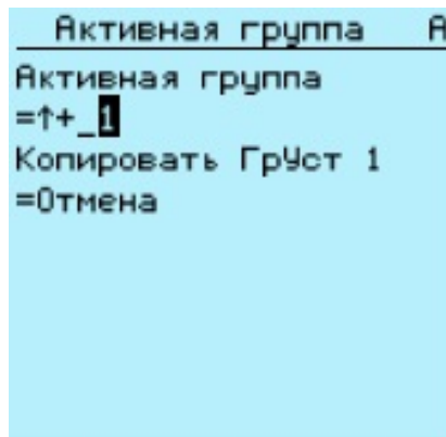
Рис. 106: Выбор активной группы уставок
