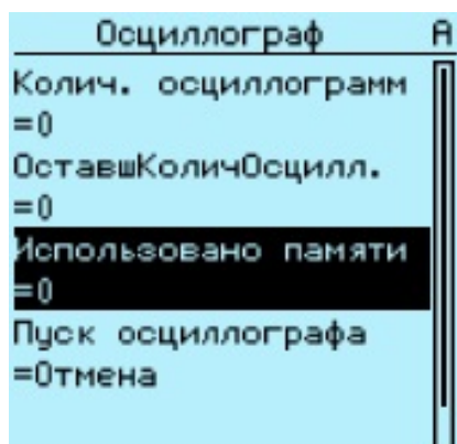
Рис. 78: Контроль данных аварийного осциллографа при помощи ЛИЧМ
