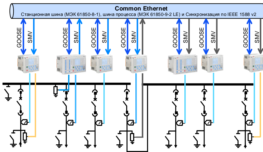
Рис. 11: Применение совместного использования напряжения и контроля синхронизма шиной процесса
