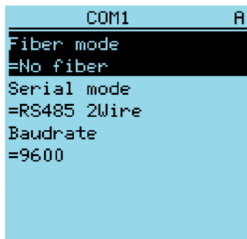
Рис. 21: Просмотр основных параметров
