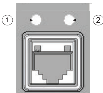
Рис. 6: Порт связи RJ-45 и светодиоды индикации
