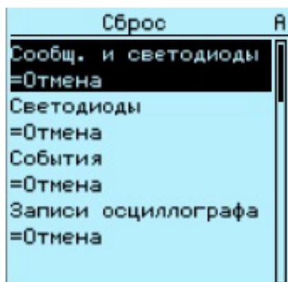
Рис. 23: Полоса прокрутки справа
