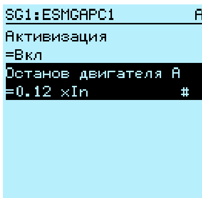
Рис. 102: Параметр группы уставок
