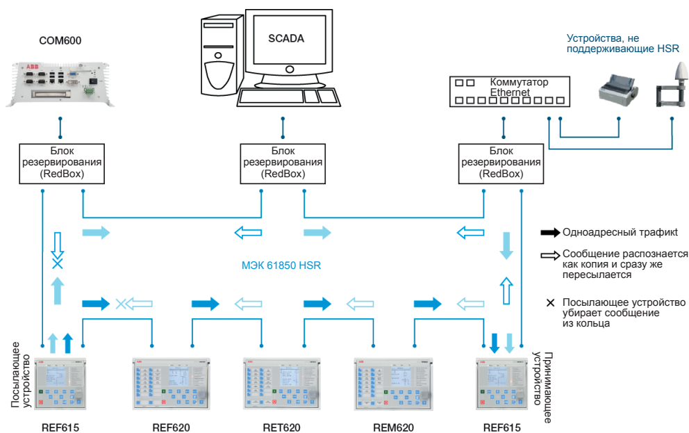
Рис. 10: Решение с использованием протокола HSR
