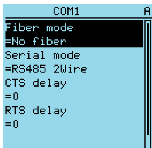
Рис. 22: Просмотр расширенного набора параметров
