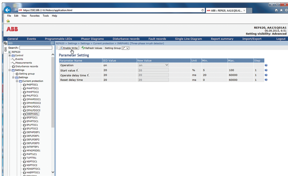
Рис. 44: Включение записи для редактирования значения
