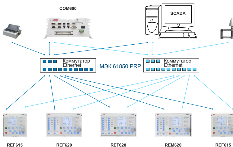
Рис. 9: Решение с использованием протокола PRP
