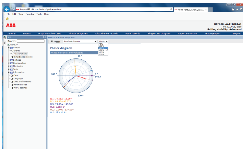
Рис. 61: Приближение диаграммы
