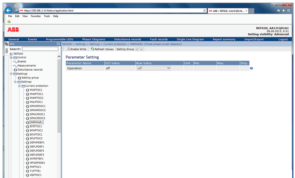
Рис. 40: Функциональный блок Выкл
