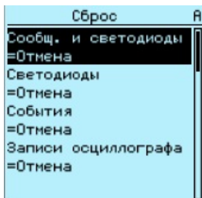
Рис. 87: Экран "Сброс"
