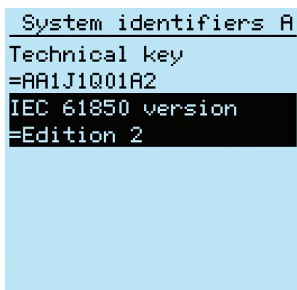
Рис. 19: Определение редакции МЭК 61850
