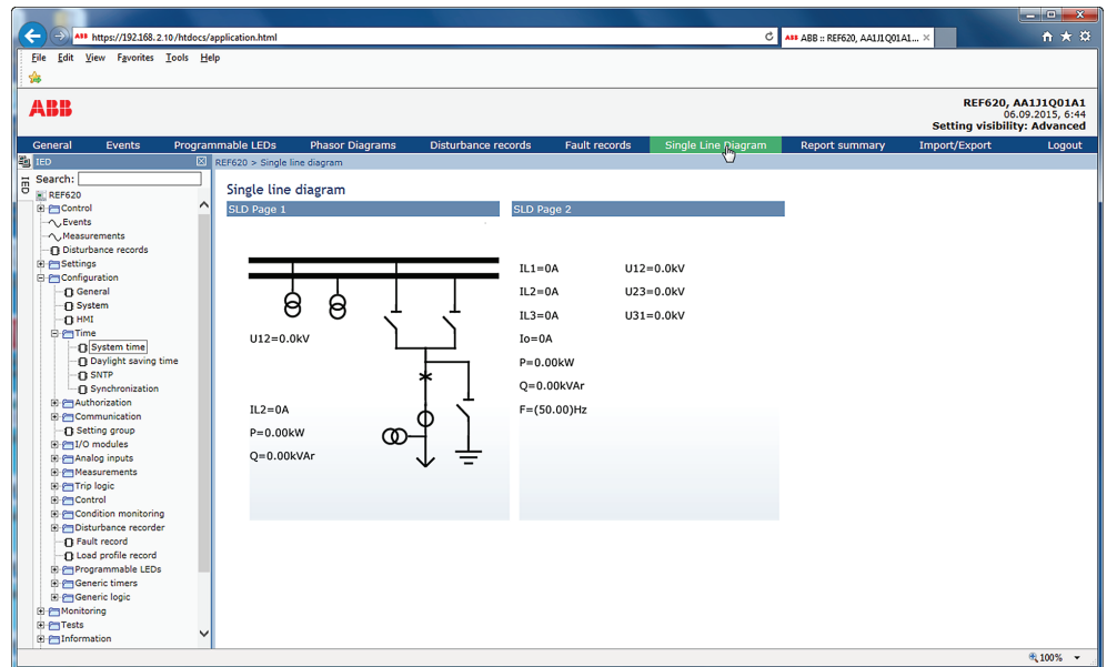
Рис. 37: Просмотр однолинейной схемы с обозначениями МЭК
