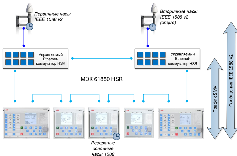
Рис. 12: Пример топологии сети с шиной процесса, резервированием и синхронизацией по IEEE 1588 v2
