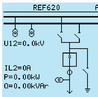
Рис. 81: Однолинейная схема с обозначениями МЭК
