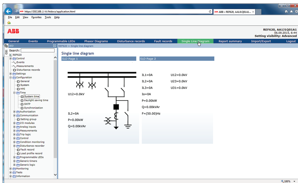
Рис. 38: Просмотр однолинейной схемы с обозначениями ANSI
