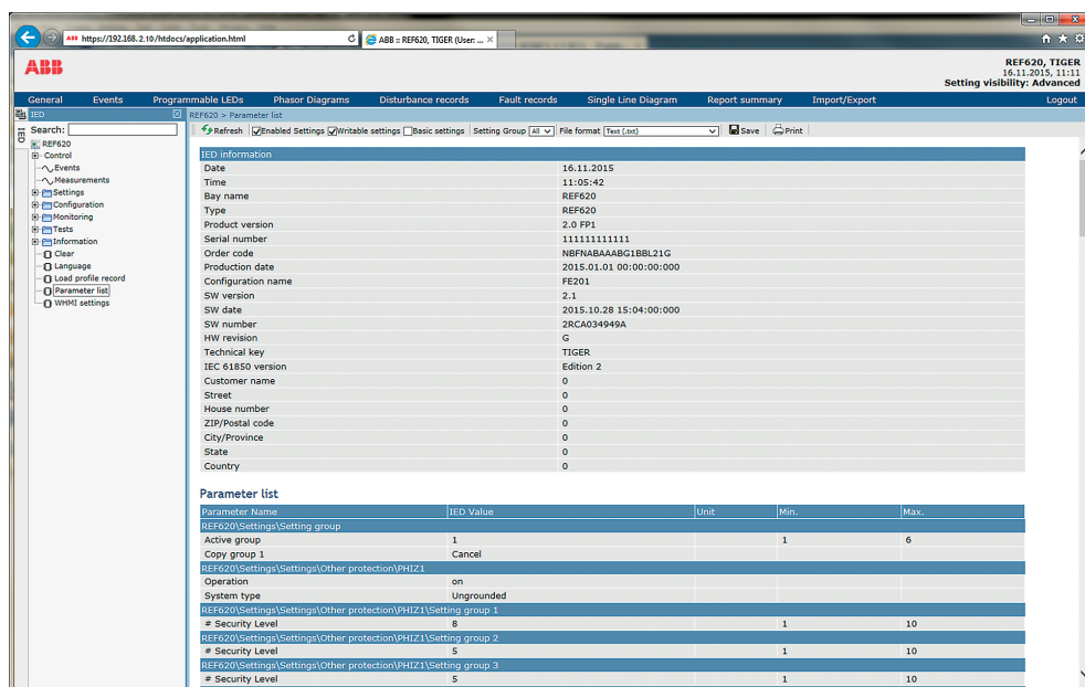
Рис. 43: Активные уставки
