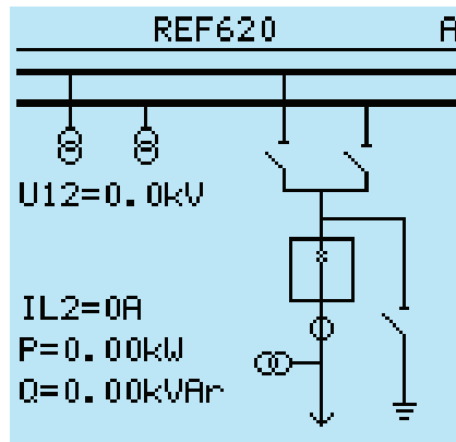
Рис. 24: Однолинейная схема с обозначениями МЭК
