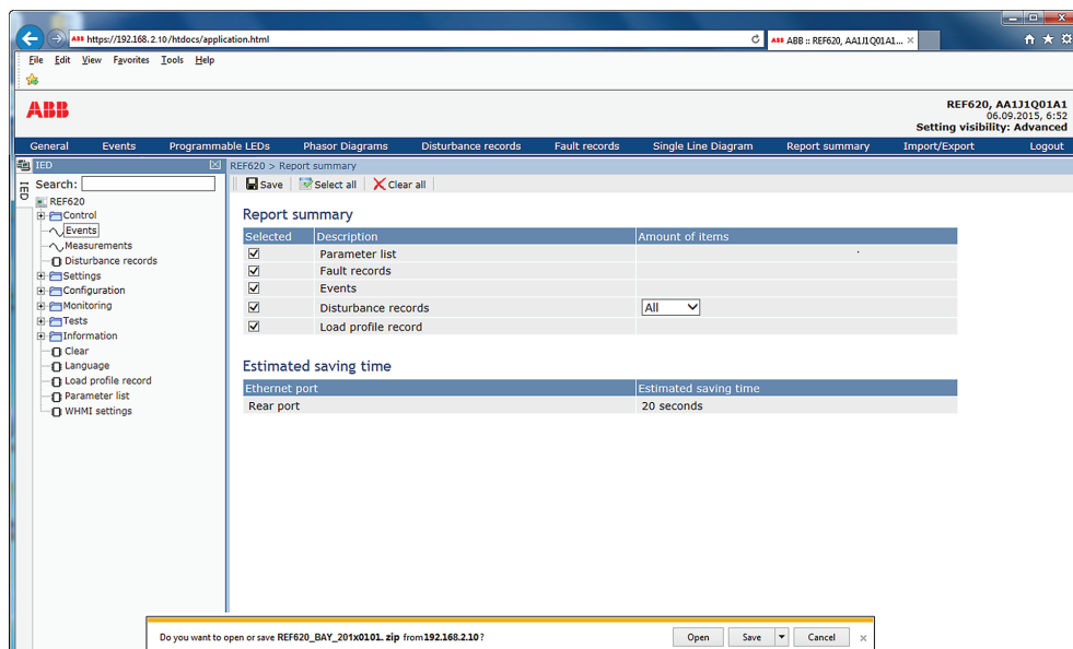
Рис. 73: Страница "Краткий отчет"
