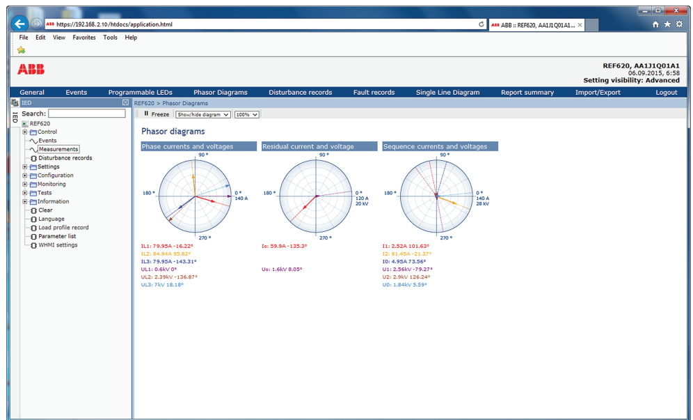
Рис. 59: Контроль векторных диаграмм
