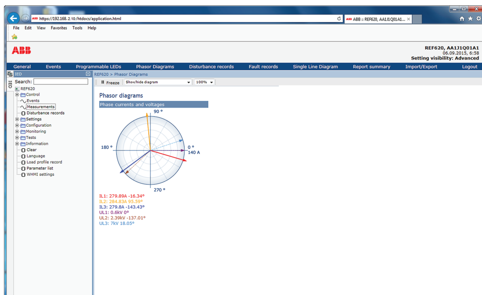
Рис. 62: Стрелка выходит за пределы окружности, если токовое значение слишком высокое
