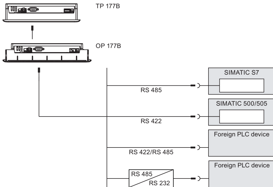
Рисунок 4-10 Подключение TP 177B или OP 177B к ПЛК
