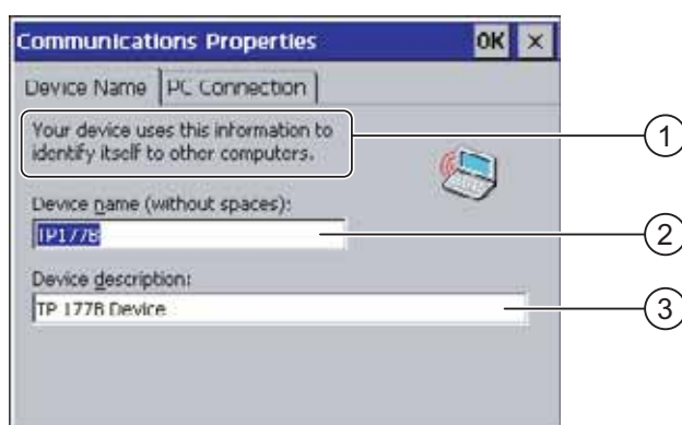
Рисунок 6-35 Диалоговое окно "Communications Properties [Настройка параметров обмена данными]", закладка "Device Name [Имя устройства]"
