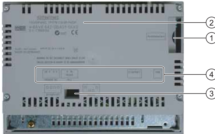
Рисунок 1-7 Вид сзади
