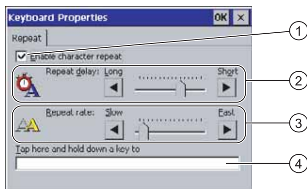
Рисунок 6-15 Диалоговое окно "Keyboard Properties [Настройка клавиатуры]"
