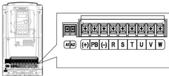
Рис. 4-11 11.5~18 кВ клеммы силовых цепей
