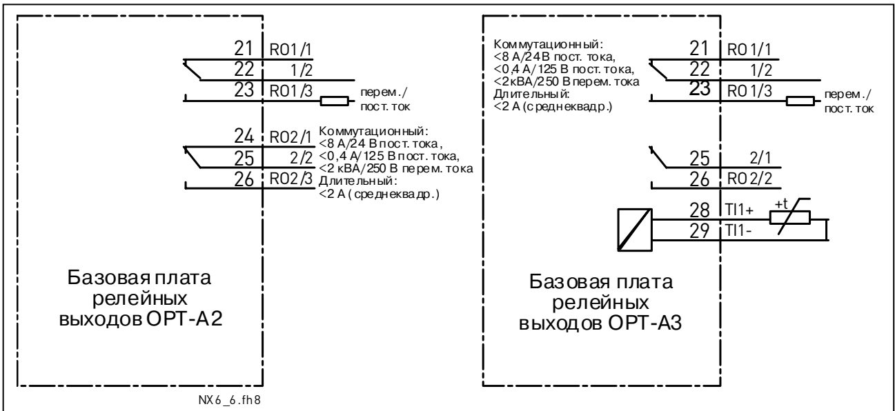
Рисунок 6-25. Принципиальная схема подсоединения базовых плат релейных выходов (OPT-A2/OPT-A3)
