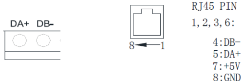
Клеммная колодка
