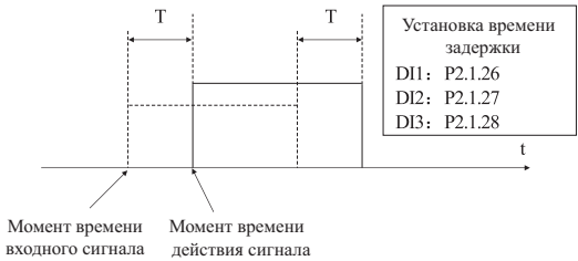
T - время задержки сигнала
