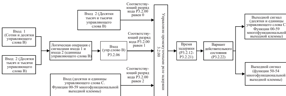
Описание функции логики управления при помощи управляющего слова V промежуточного реле задержки
