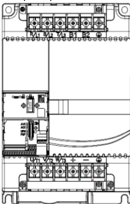
Типоразмер D
