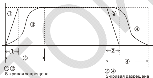
Характеристики разгона/торможения
