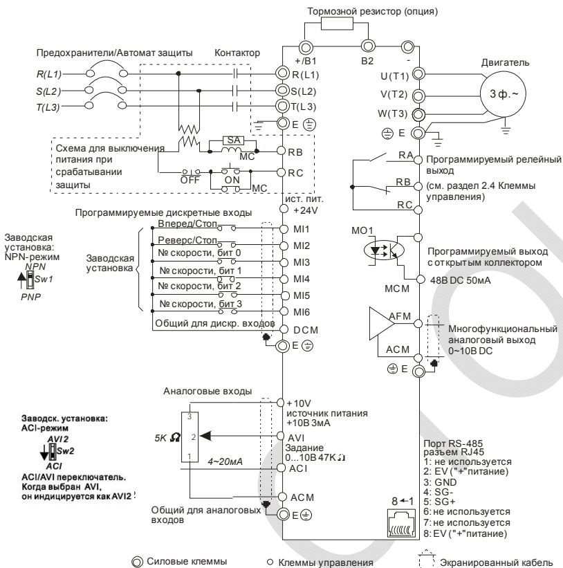
Рисунок 4. Схема для моделей VFD022E23A/43A, VFD037E23A/43A, VFD055E23A/43A, VFD075E23A/43A, VFD110E23A/43A, VFD022E23C/43C, VFD037E23C/43C, VFD055E23C/43C, VFD075E23C/43C, VFD110E23C/43C, VFD150E23A/23C, VFD150E43A/43C, VFD185E43A/43C, VFD220E43A/43C
