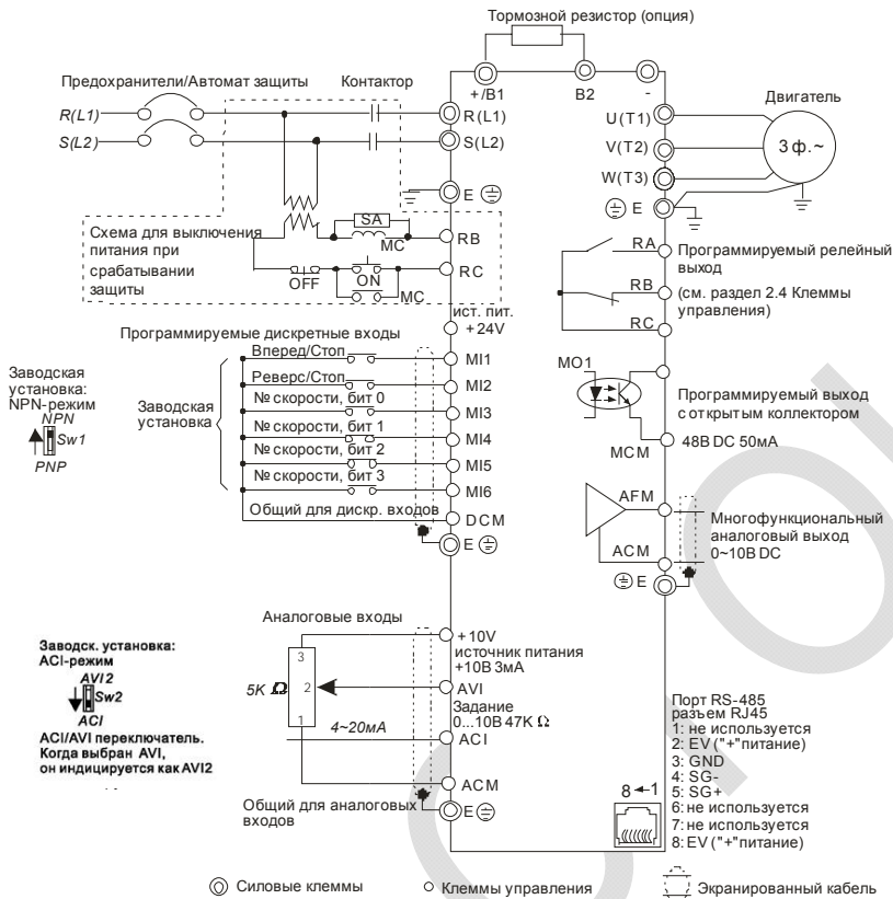
Рисунок 3. Схема для моделей VFD007E11A, VFD015E21A, VFD022E21A, VFD0 0E 11C VFD015E21C, VFD022E21C
