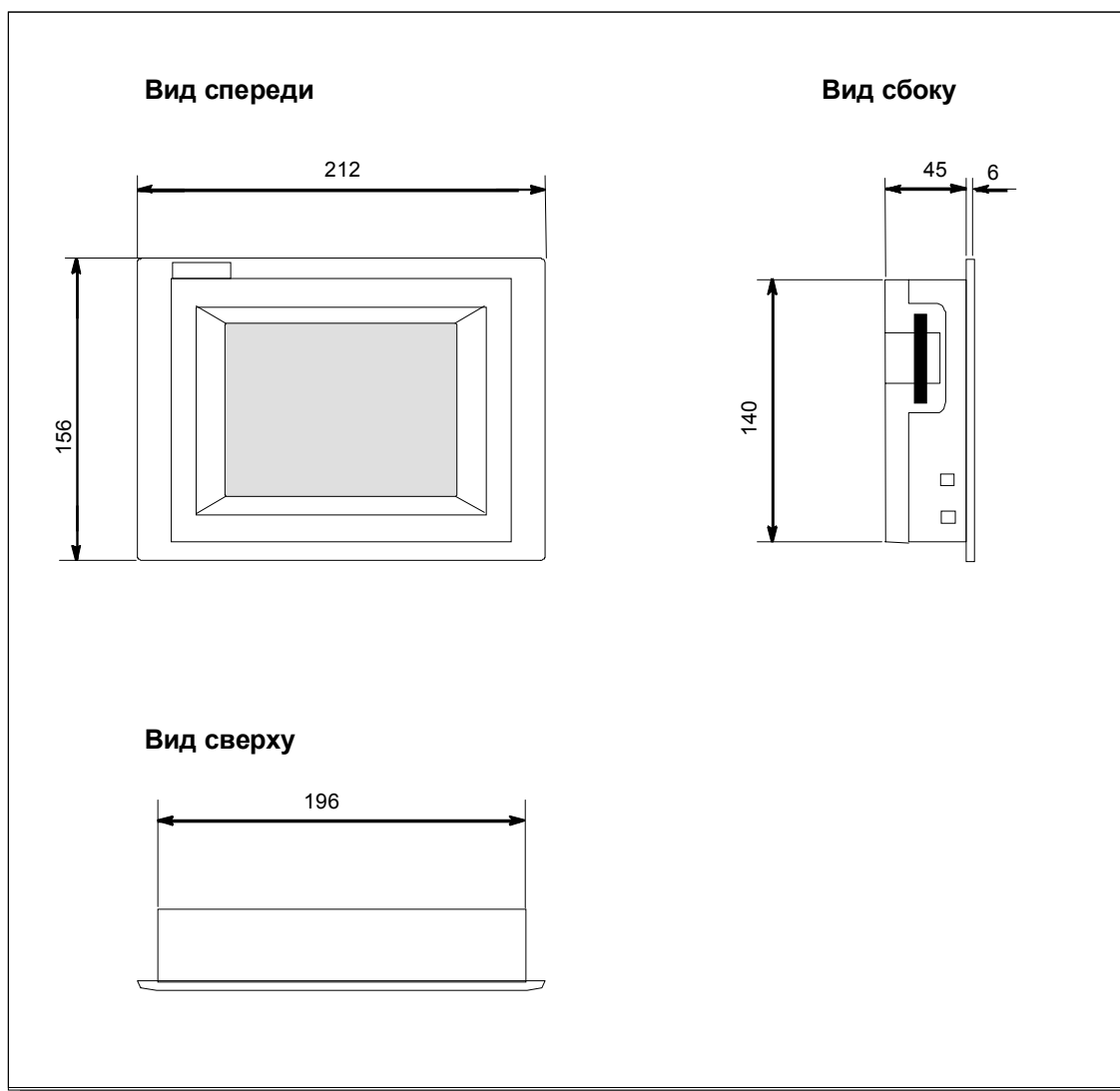
Рис. 9–1. Размеры TP 070
