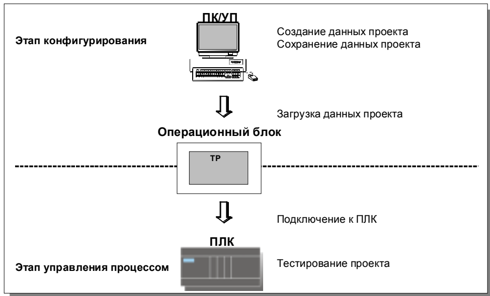
Рис. 1-1. Этапы конфигурирования и управления процессом
