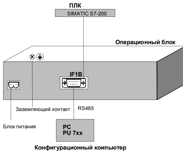
Рис. 8–1. Возможности конфигурирования
