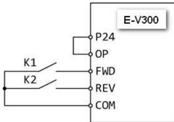
Двухпроводный режим
