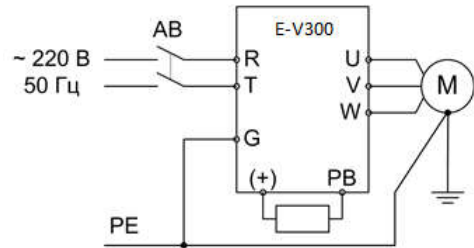
Подключение ПЧ 220 В 0,75...2,2 кВт с тормозным резистором
