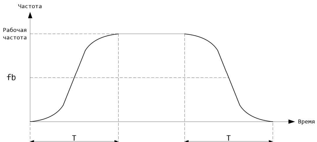
График S-образной зависимости разгона / торможения Б
