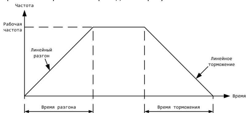
Профиль разгона / торможения
