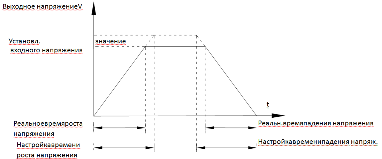
Схема разделения V/f
