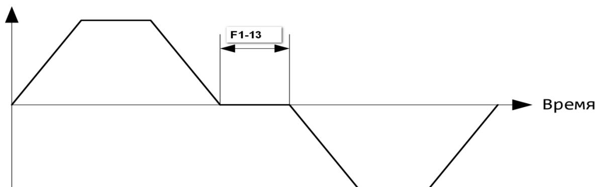
Пауза при смене направления вращения
