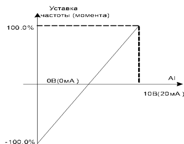
График зависимости частоты (момента) от сигнала на аналоговых входах при использовании характеристики 5
