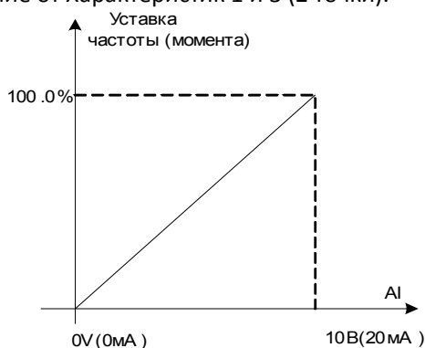
График зависимости частоты (момента) от сигнала на аналоговых входах при использовании характеристики 4
