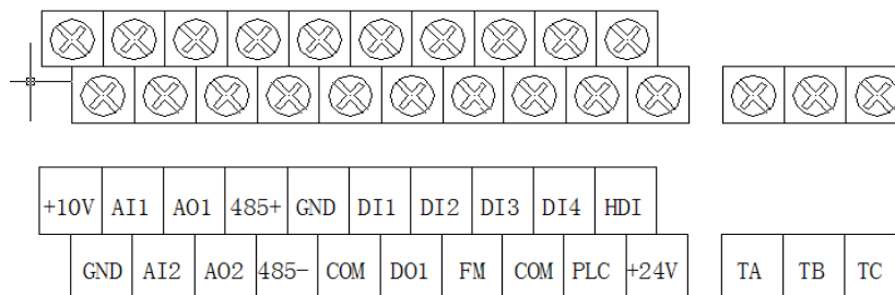
Схема расположения клемм на ПЧ
