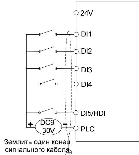
Подключение входов типа «открытый коллектор PNP» с внешним источником питания +24В
