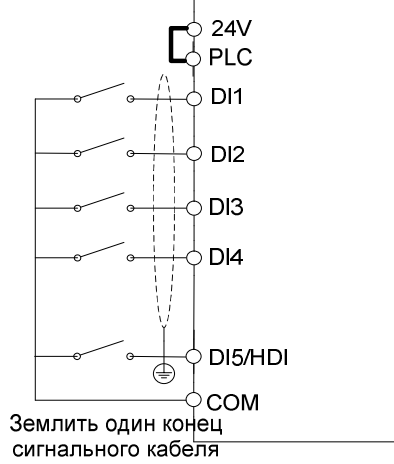
Подключение входов типа «открытый коллектор NPN» со встроенным источником питания +24В
