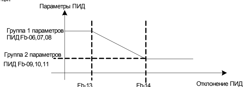
График переключения параметра ПИД
