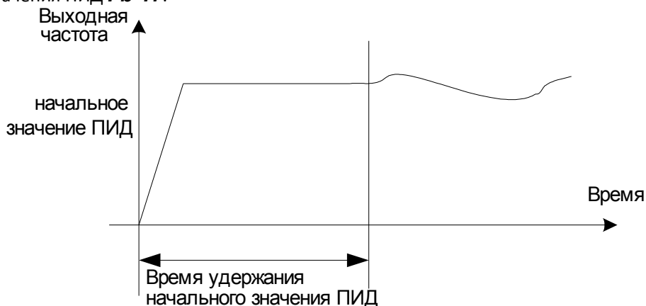
Функция начального значения ПИД
