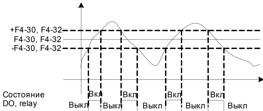
Определение порогов выходного тока ПЧ
