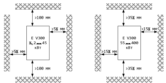
Установка ПЧ в шкафу
