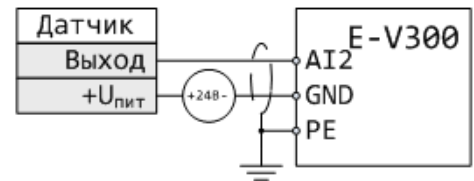
Типовые схемы подключения аналоговых входов AI1, AI2
