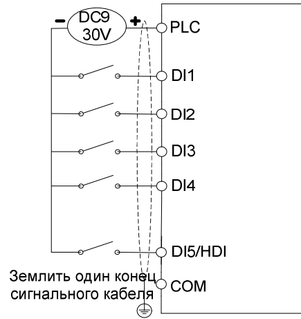
Подключение входов типа «открытый коллектор NPN» с внешним источником питания +24В
