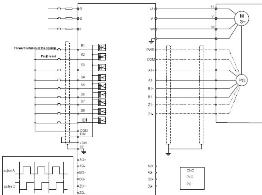
Рис. 4-26 Схема подключения EC-PG305-12
