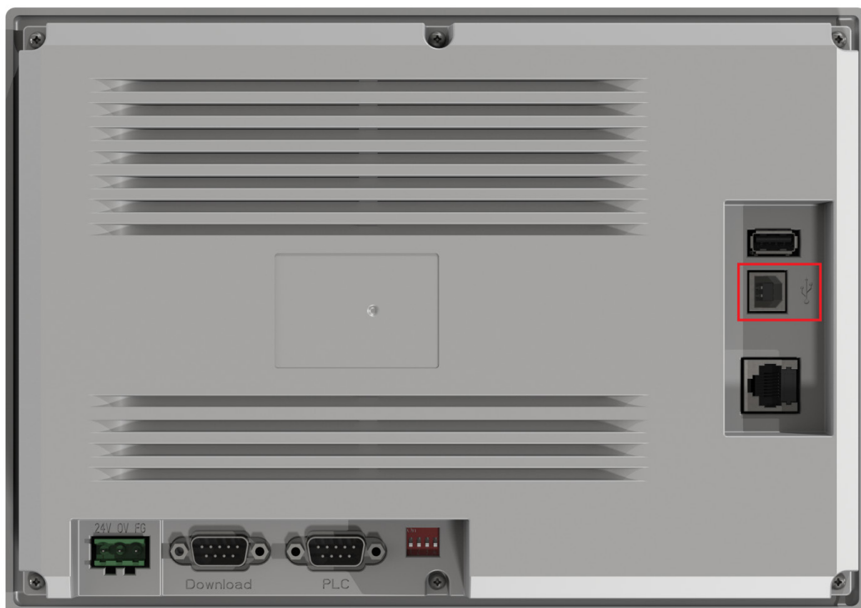
Рисунок 6.1 – Внешний вид задней крышки панели СП3хх-Р (порт USB В обведен красным)
