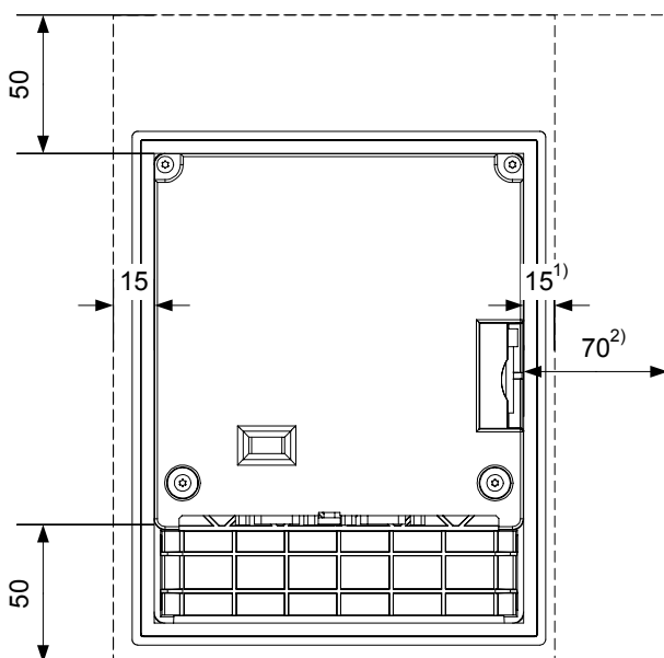
Рисунок 3-6 Зазоры между ОР 77А и ОР 77В и монтажным вырезом
