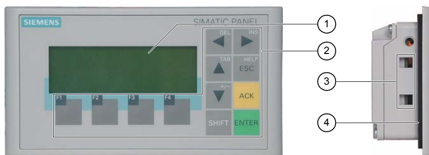
Рисунок 1-1 Фронтальный и боковой виды
