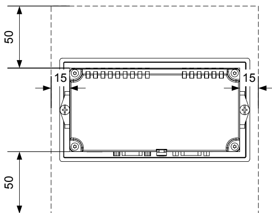
Рисунок 3-5 Зазоры между ОР 73 и монтажным вырезом
