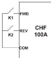
Рисунок 6.11. Двухпроводное управление режим 1.
