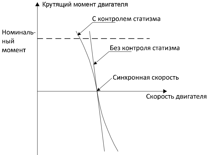
Рисунок 6.23. Контроль статизма.
