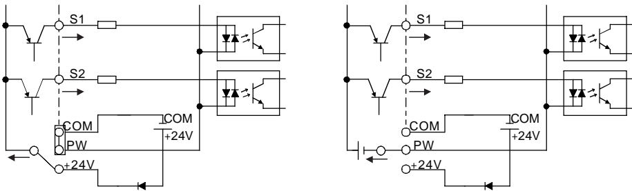
Режим с общим эмиттером (+24В общий) для внутр. питания Режим с общим эмиттером (+24В общий) для внеш. питания
