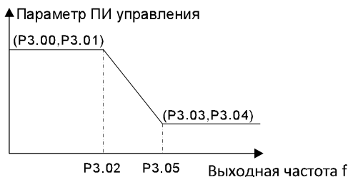
Рисунок 6.7. Диаграмма параметров PI управления
