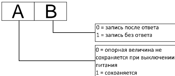
Рисунок 6.36. Значение PC.06.
