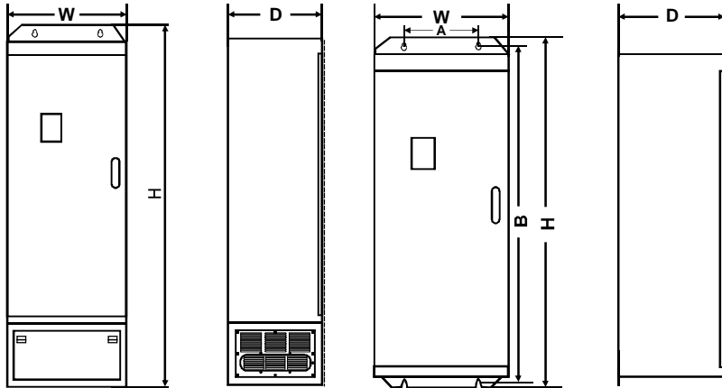
Рисунок А. 3. Габаритные размеры (132–500кВт)
