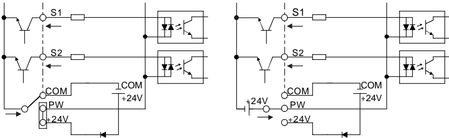
Режим с общим эмиттером (0В общий) для внутр. питания
