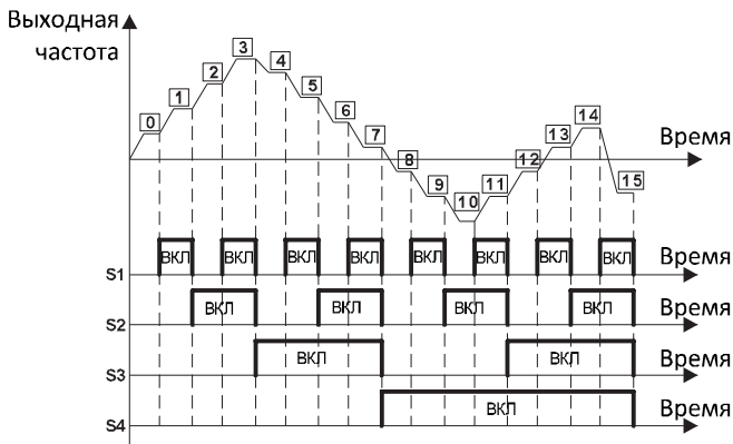
Рисунок 6.30. Схема многоступенчатого регулирования скорости.
