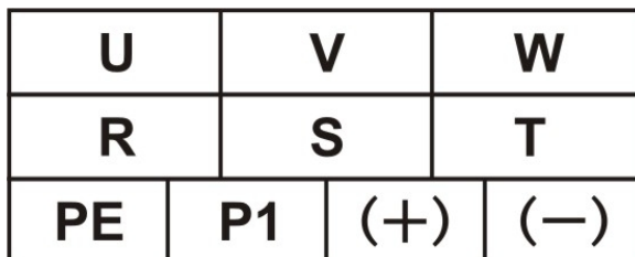
Рисунок 4.6. Клеммы силовой цепи (350–630 кВт)
