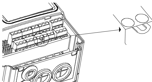
Рисунок 4.13. U-образная перемычка.
