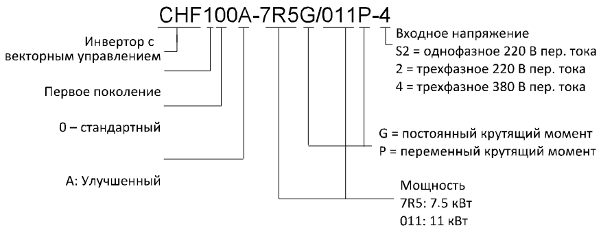
Рисунок 1.1. Расшировка номера инвертора
