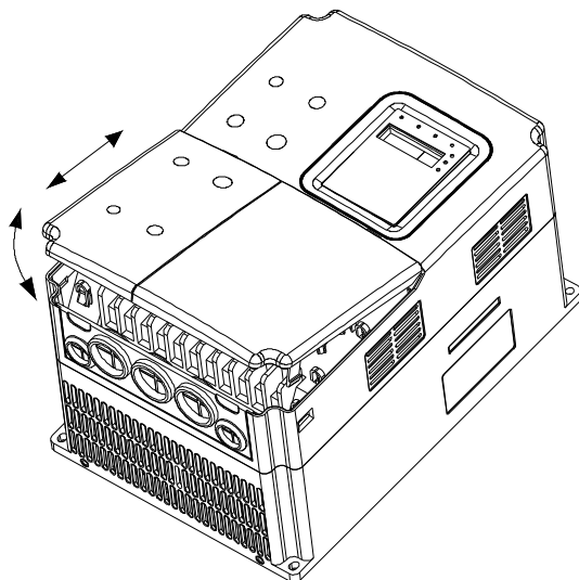
Рисунок А. 13. Снятие пластиковой крышки
