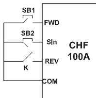
Рисунок 6.13. Трехпроводное управление режим 1.
