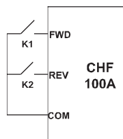
Рисунок 6.12. Двухпроводное управление режим 2.
