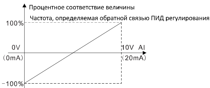
Рисунок 6.15. Отношение между сигналом аналогового входа AI и соответствующей величиной.
