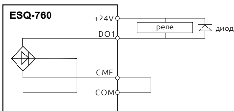
Рисунок 3-22. Схема подключения реле к выходу DO1.
