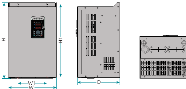
Рисунок 2-7. Установочные размеры ПЧ мощностью до 11-45 кВт
