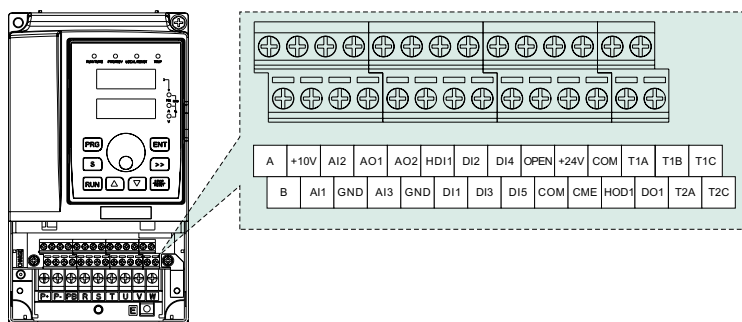
Рисунок 3-17. Клеммы управления.
