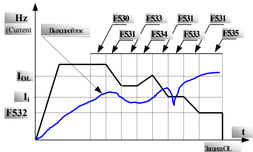
Рис.9-3 Настройка торможения
