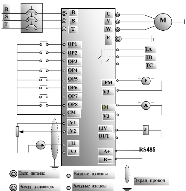
Рис.3-3 Схема подключения трёхфазного инвертора
