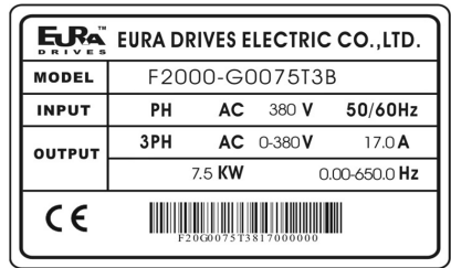
Рис.1-1 Иллюстрация шильдика
