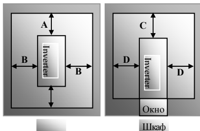
Рис.3-1 Установка
