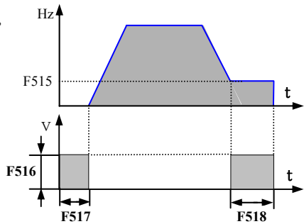
Рис.9-2 Торможение
