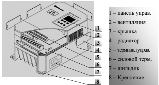
Рис. 1-3 Внешний вид пластикового корпуса
