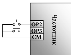
Рис.3-4 Трёхлинейная схема
