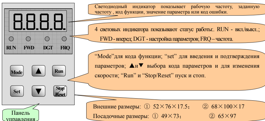
Рис.2-1 Панель управления двух типов
